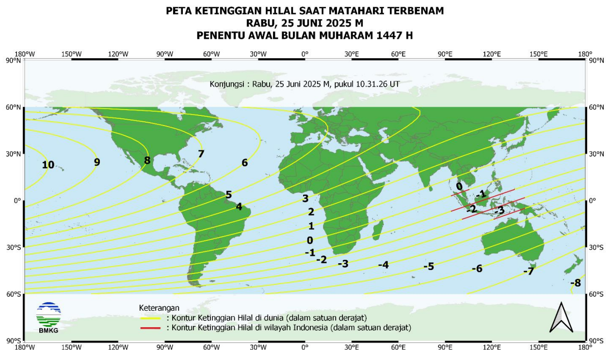
Gambar 1. Peta ketinggian Hilal tanggal 25 Juni 2025 untuk pengamat antara 60^\circ LU sampai dengan 60^\circ LS
