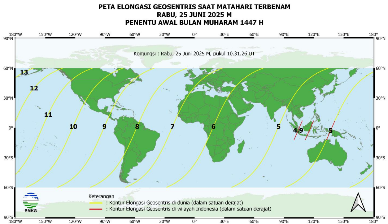
Gambar 5. Peta elongasi geosentris tanggal 25 Juni 2025 untuk pengamat antara 60° LU sampai dengan 60° LS
