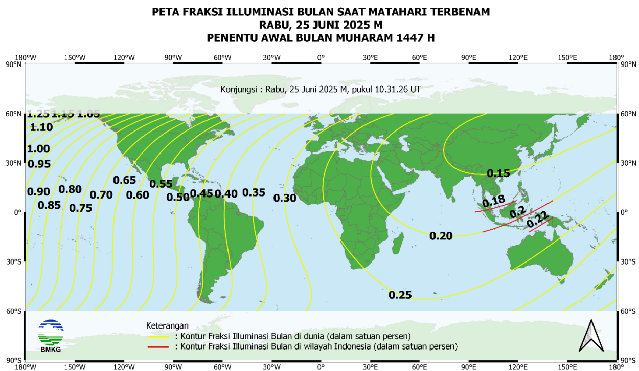
Gambar 17. Peta fraksi iluminasi bulan tanggal 25 Juni 2025 untuk pengamat antara 60^\circ LU s.d. 60^\circ LS
