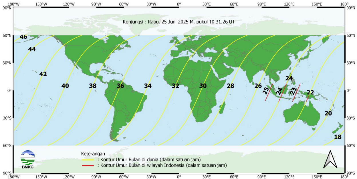
Gambar 11. Peta umur bulan tanggal 26 Juni 2025 untuk pengamat antara 60° LU sampai dengan 60° LS
