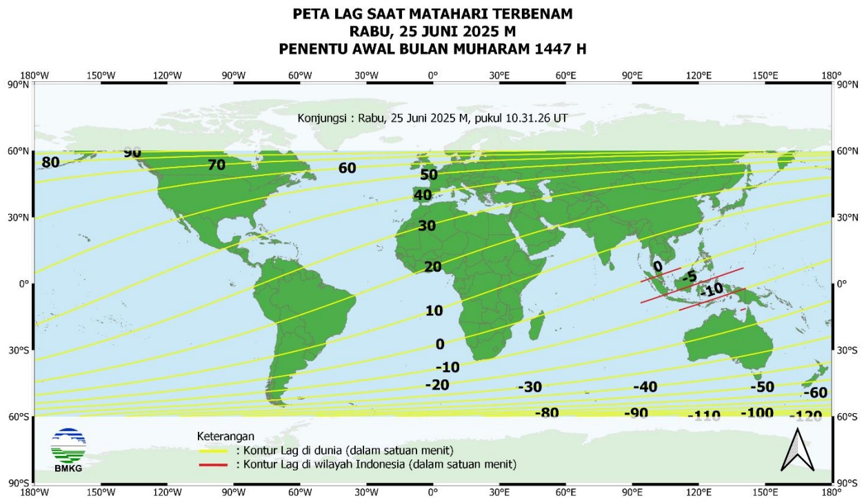
Gambar 13. Peta lag tanggal 25 Juni 2025 untuk pengamat antara 60° LU sampai dengan 60° LS
