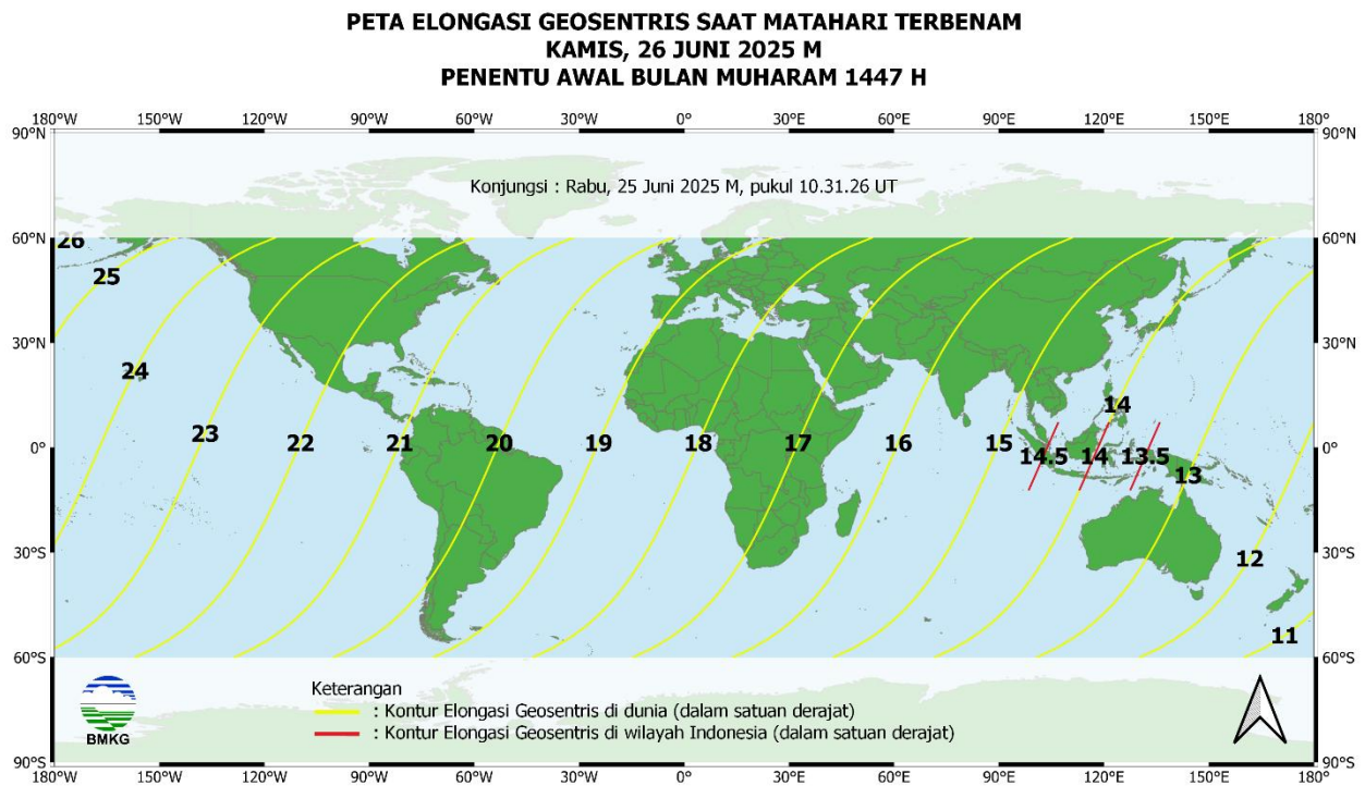
Gambar 7. Peta elongasi geosentris tanggal 26 Juni 2025 untuk pengamat antara 60° LU sampai dengan 60° LS
