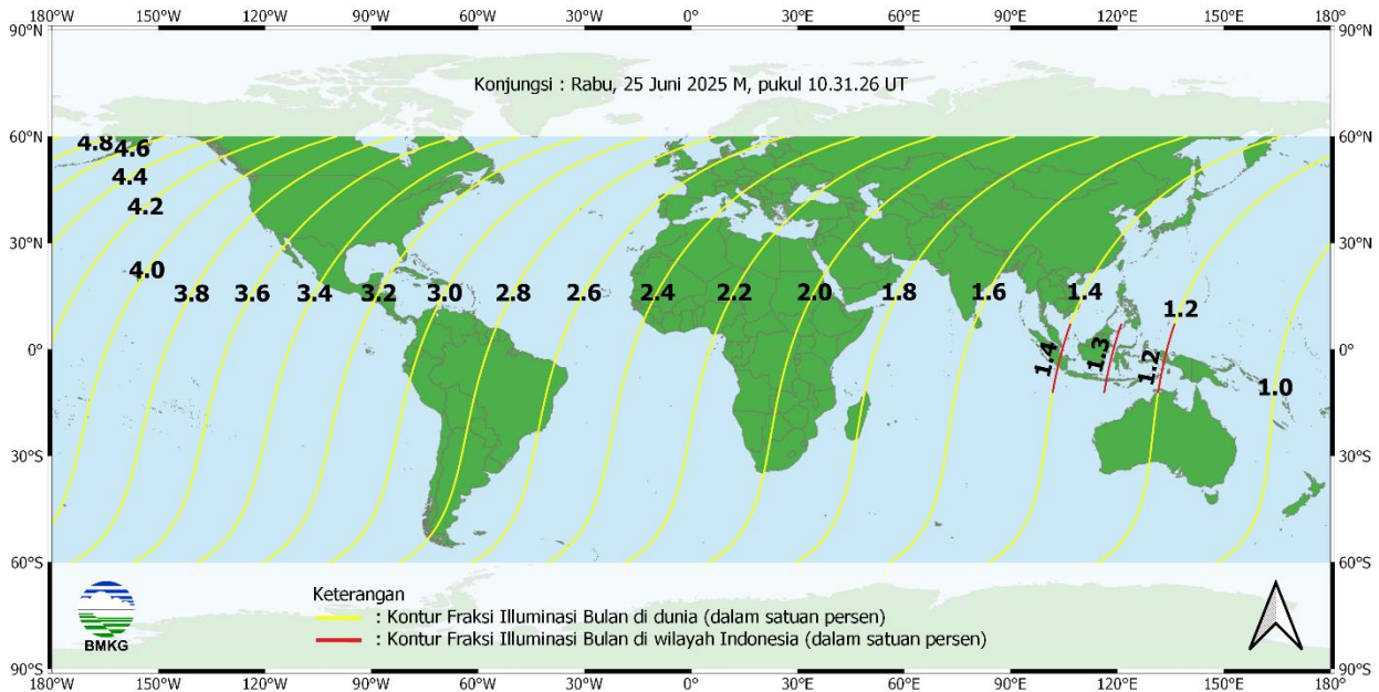
Gambar 19. Peta fraksi illuminasi bulan tanggal 26 Juni 2025 untuk pengamat antara 60° LU s.d. 60° LS
