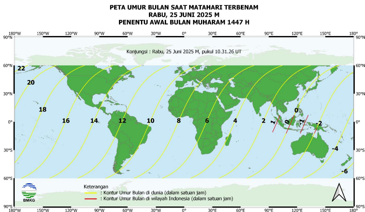
Gambar 9. Peta umur bulan tanggal 25 Juni 2025 untuk pengamat antara 60^\circ LU sampai dengan 60^\circ LS
