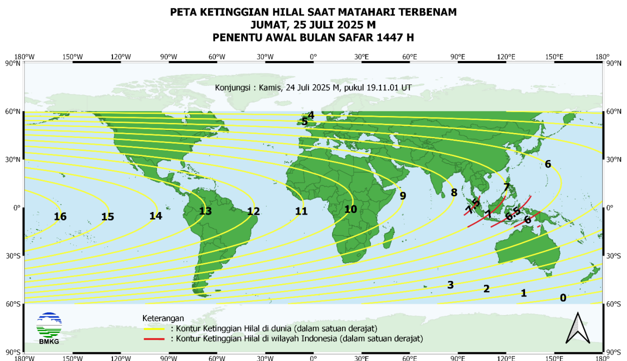
Gambar 1. Peta ketinggian Hilal tanggal 25 Juli 2025 untuk pengamat antara 60^\circ LU sampai dengan 60^\circ LS
