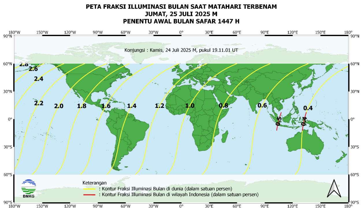
Gambar 9. Peta fraksi iluminasi bulan tanggal 25 Juli 2025 untuk pengamat antara 60° LU s.d. 60° LS
