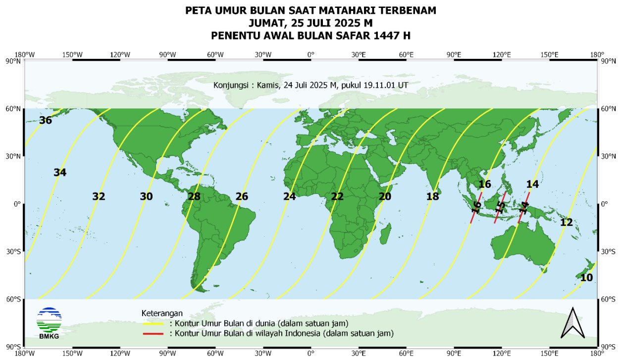
Gambar 5. Peta umur bulan tanggal 25 Juli 2025 untuk pengamat antara 60° LU sampai dengan 60° LS
