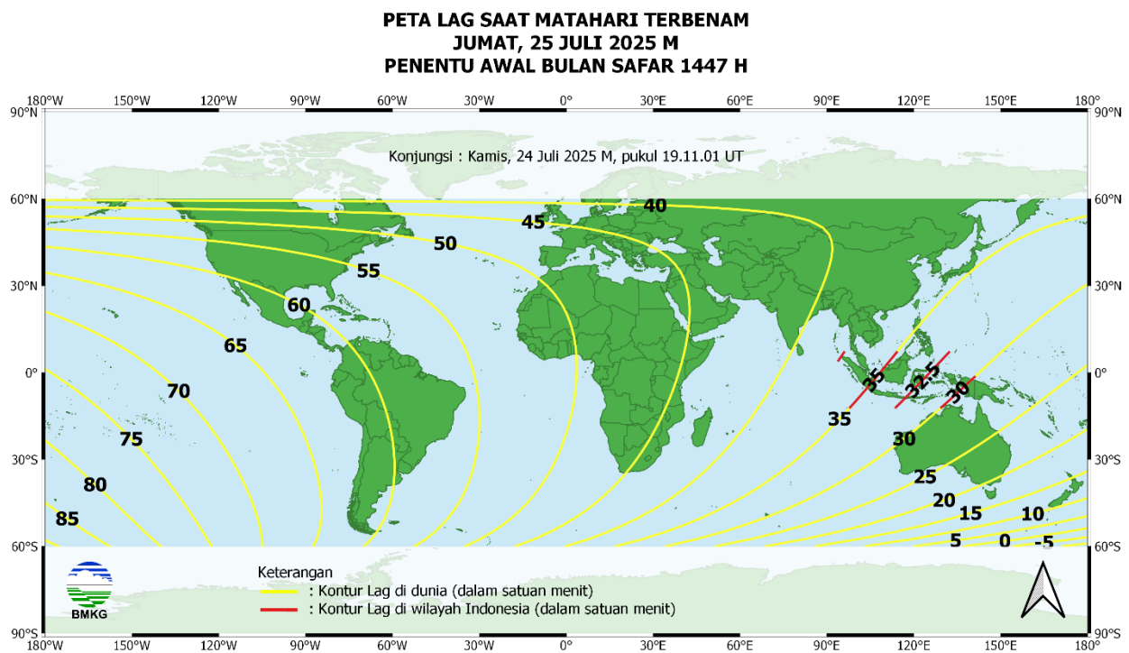
Gambar 7. Peta lag tanggal 25 Juli 2025 untuk pengamat antara 60° LU sampai dengan 60° LS
