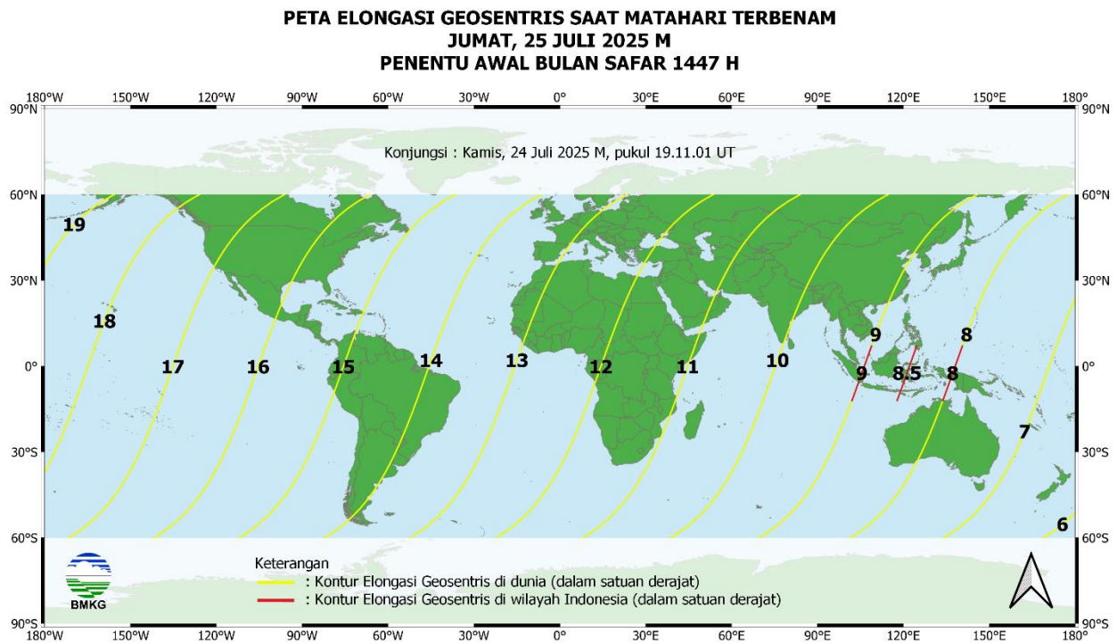
Gambar 3. Peta elongasi geosentris tanggal 25 Juli 2025 untuk pengamat antara 60° LU sampai dengan 60° LS
