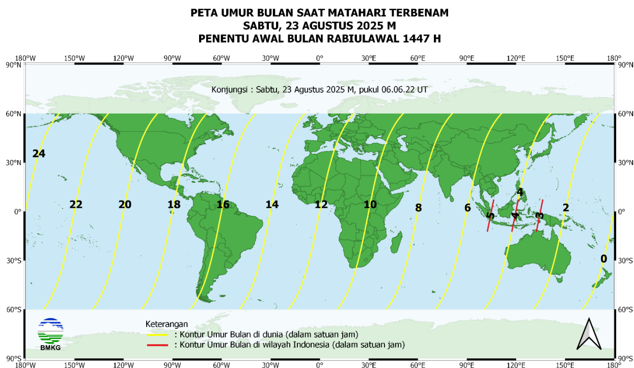
Gambar 9. Peta umur bulan tanggal 23 Agustus 2025 untuk pengamat antara 60^\circ LU sampai dengan 60^\circ LS
