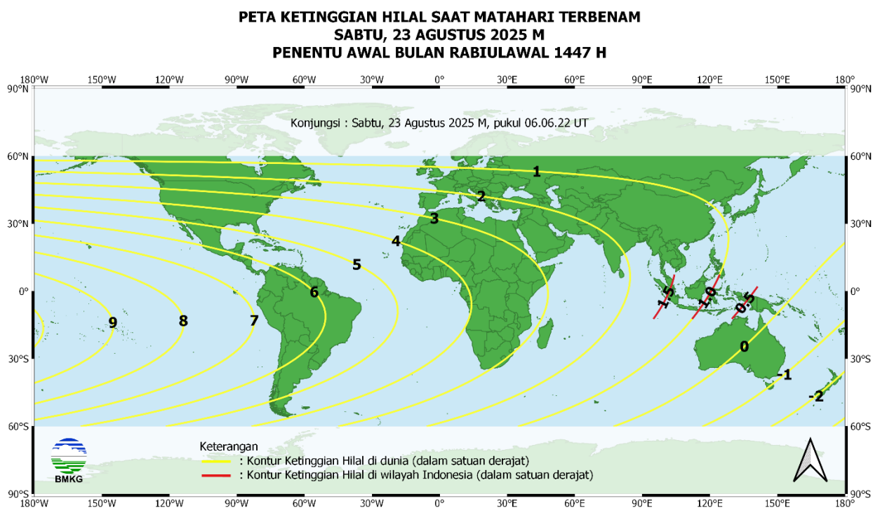
Gambar 1. Peta ketinggian Hilal tanggal 23 Agustus 2025 untuk pengamat antara 60^\circ LU sampai dengan 60^\circ LS
