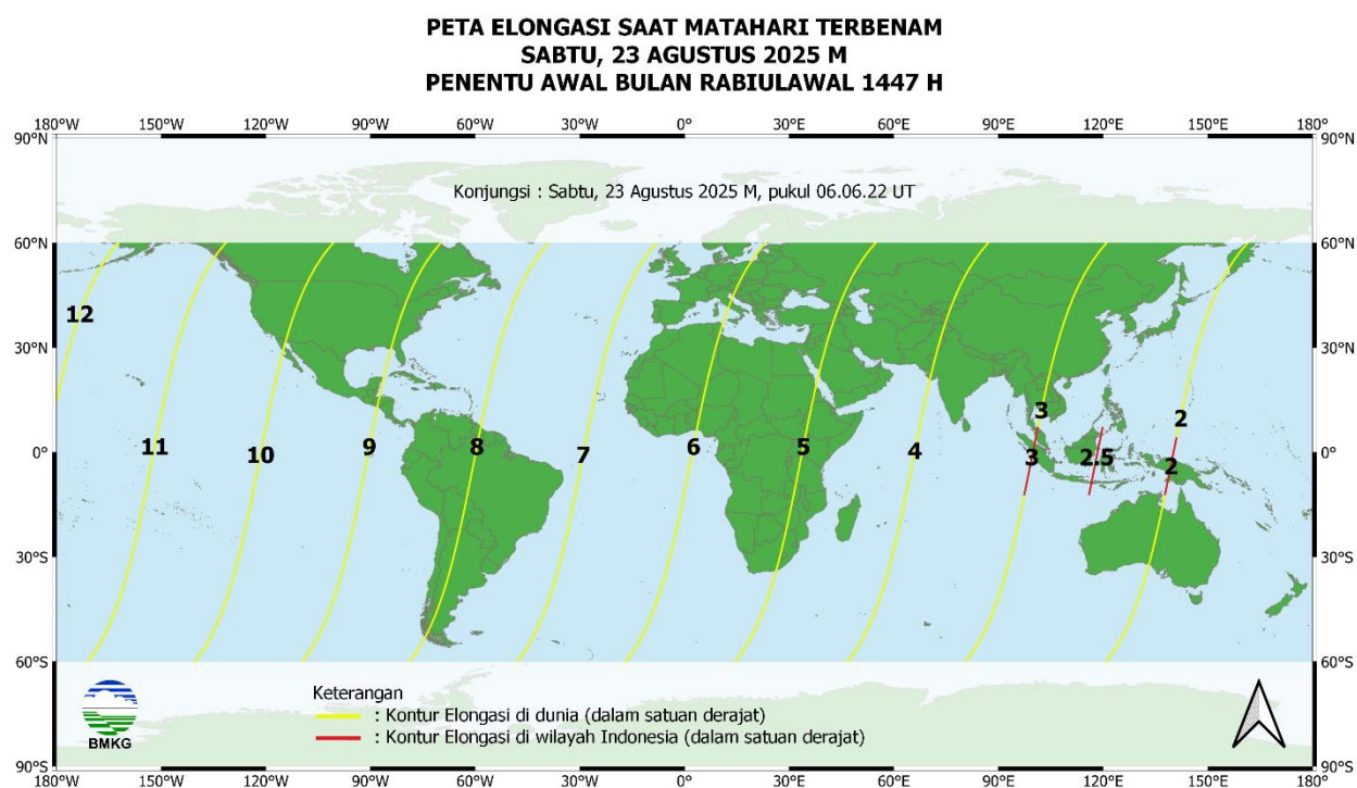
Gambar 5. Peta elongasi geosentris tanggal 23 Agustus 2025 untuk pengamat antara 60° LU sampai dengan 60° LS
