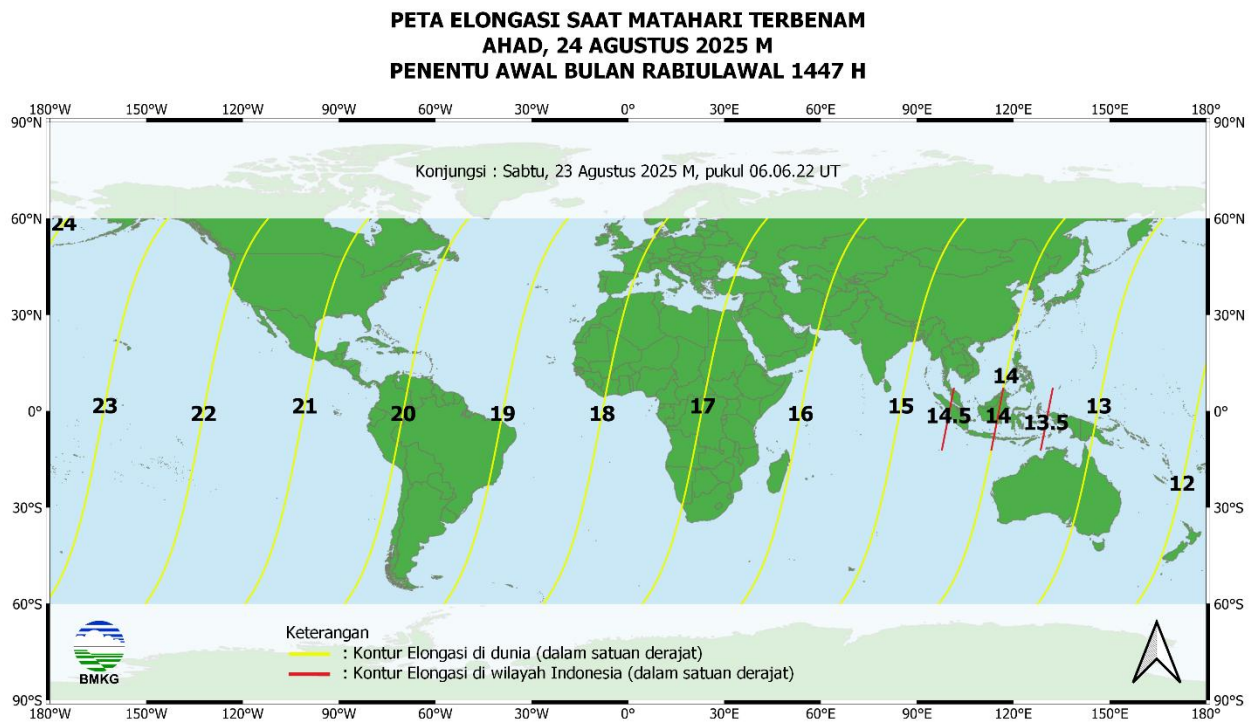
Gambar 7. Peta elongasi geosentris tanggal 24 Agustus 2025 untuk pengamat antara 60° LU sampai dengan 60° LS
