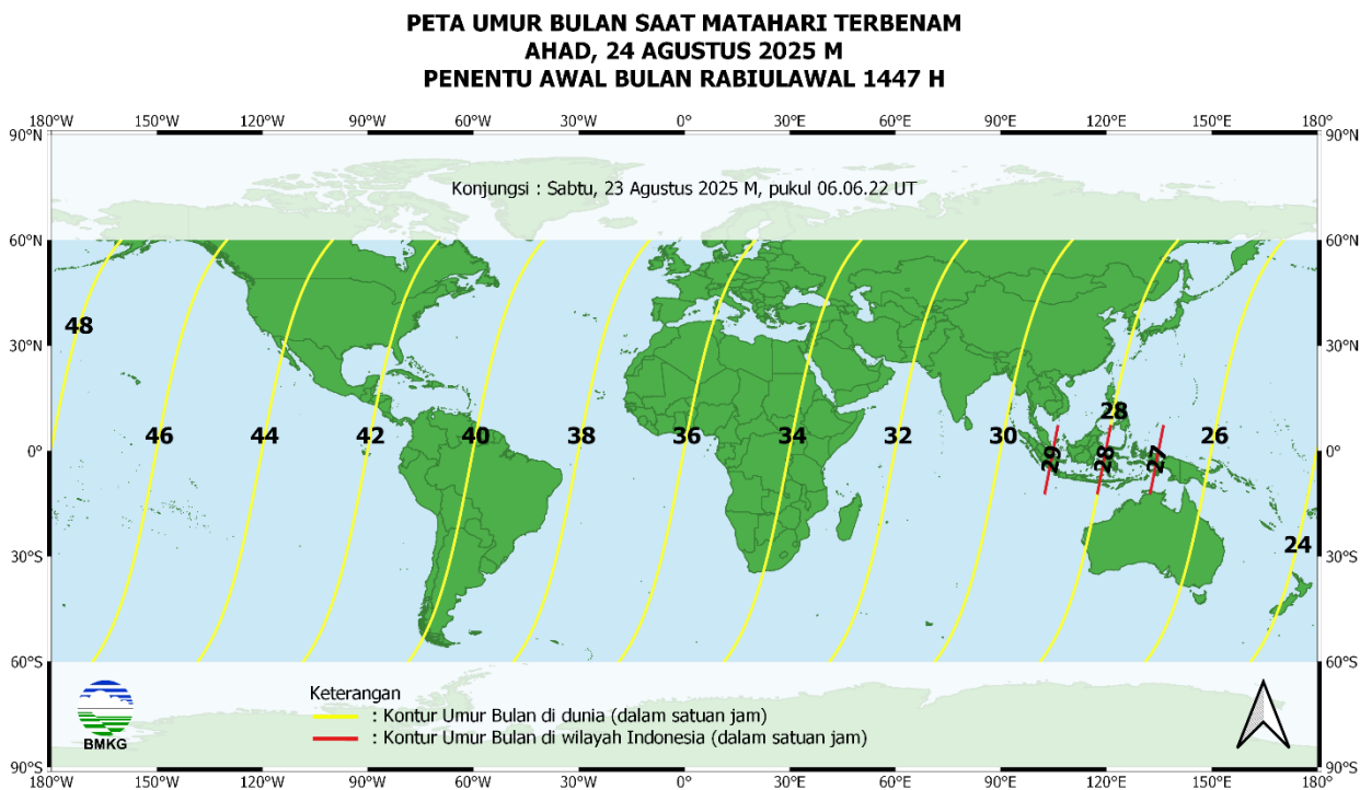
Gambar 11. Peta umur bulan tanggal 24 Agustus 2025 untuk pengamat antara 60° LU sampai dengan 60° LS
