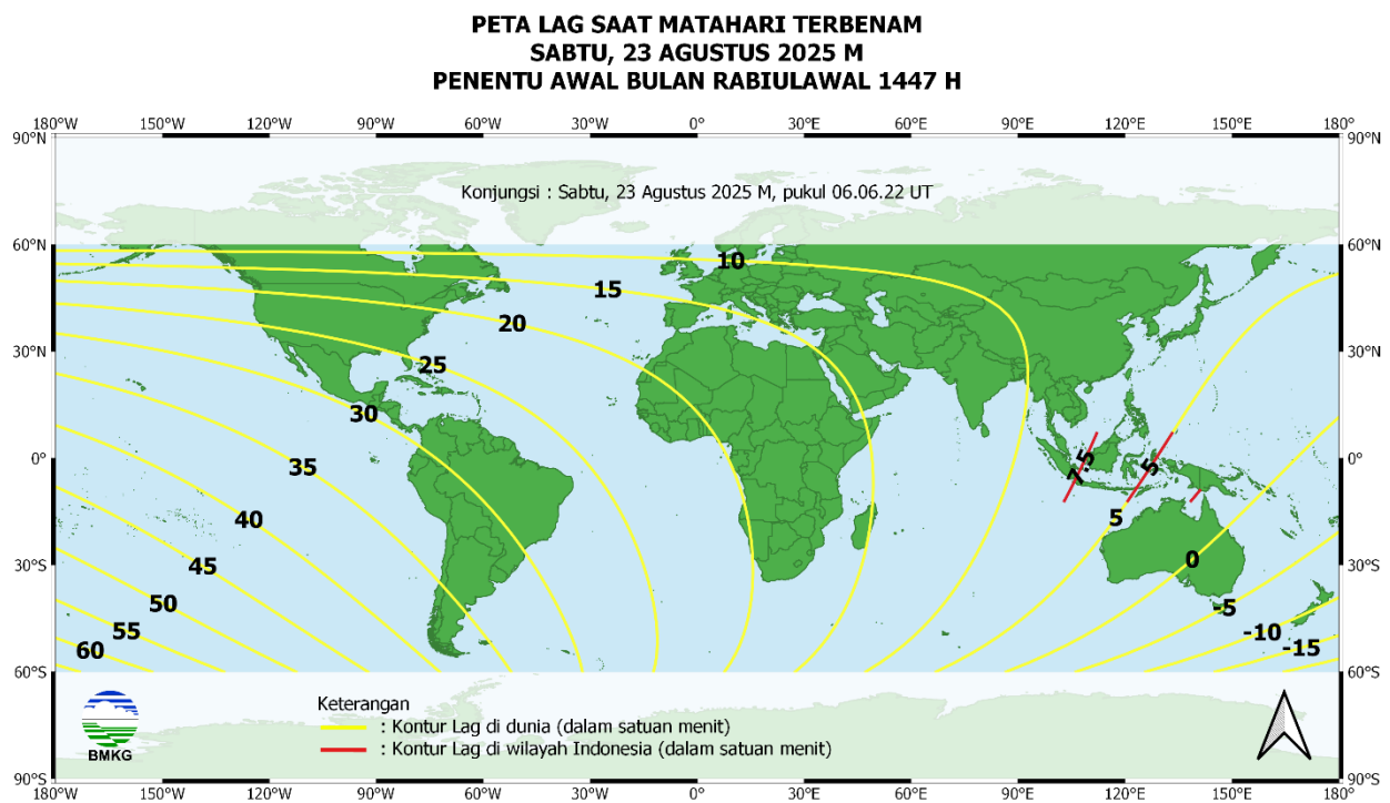
Gambar 13. Peta lag tanggal 23 Agustus 2025 untuk pengamat antara 60° LU sampai dengan 60° LS
