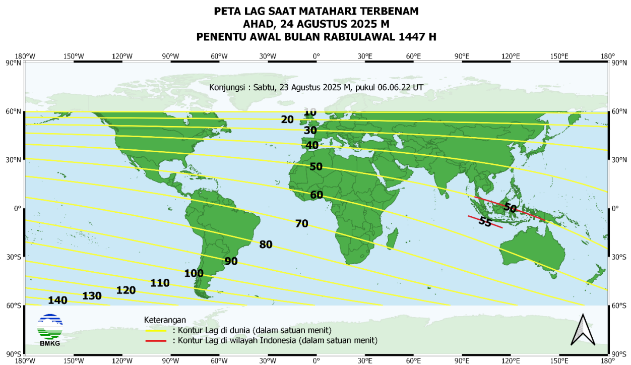
Gambar 15. Peta lag tanggal 24 Agustus 2025 untuk pengamat antara 60° LU sampai dengan 60° LS
