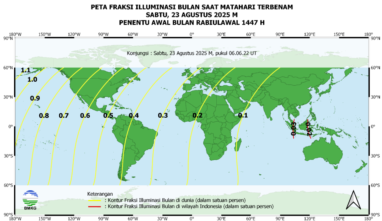
Gambar 17. Peta fraksi iluminasi bulan tanggal 23 Agustus 2025 untuk pengamat antara 60^\circ LU s.d. 60^\circ LS
