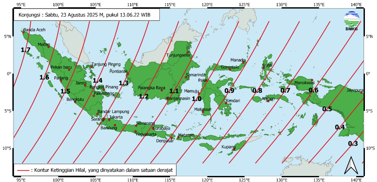
Gambar 2. Peta ketinggian Hilal tanggal 23 Agustus 2025 untuk pengamat di Indonesia
